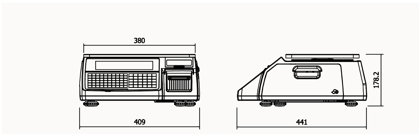
Рисунок 1.2 – Вид весов CL3000-B в геометрической проекции
