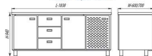
СШС-3,2-1850 / СШН-3,2-1850
