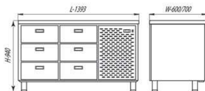
СШС-6,0-1400 / СШН-6,0-1400
