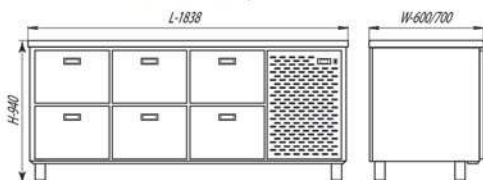
СШС-6,0-1850 / СШН-6,0-1850
