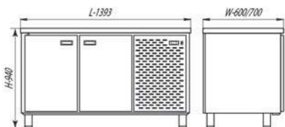
СШС-0,2-1400 / СШН-0,2-1400
