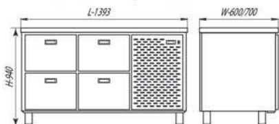
СШС-4,0-1400 / СШН-4,0-1400
