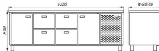
СШС-4,2-2300 / СШН-4,2-2300
