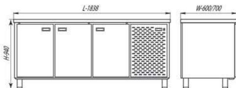
СШС-0,3-1850 / СШН-0,3-1850
