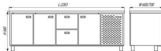
СШС-2,3-2300 / СШН-2,3-2300
