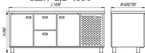
СШС-2,2-1850 / СШН-2,2-1850
