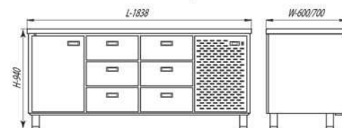
СШС-6,1-1850 / СШН-6,1-1850
