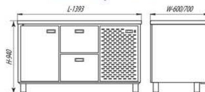
СШС-2,1-1400 / СШН-2,1-1400
