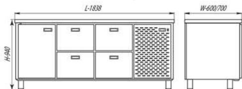
СШС-4,1-1850 / СШН-4,1-1850
