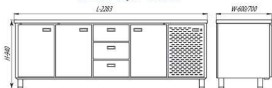
СШС-3,3-2300 / СШН-3,3-2300
