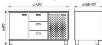
СШС-3,1-1400 / СШН-3,1-1400
